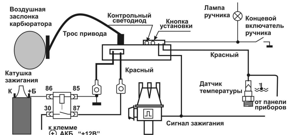
Рисунок 1 – Схема подключения устройства
